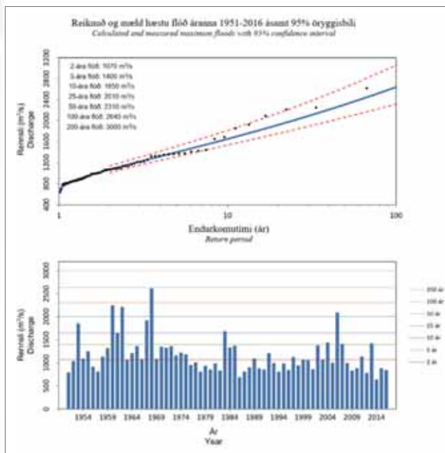
Mynd 1. Reiknuð og mæld hæstu flóð við vatnshæðarmæli 064 við Selfoss.
